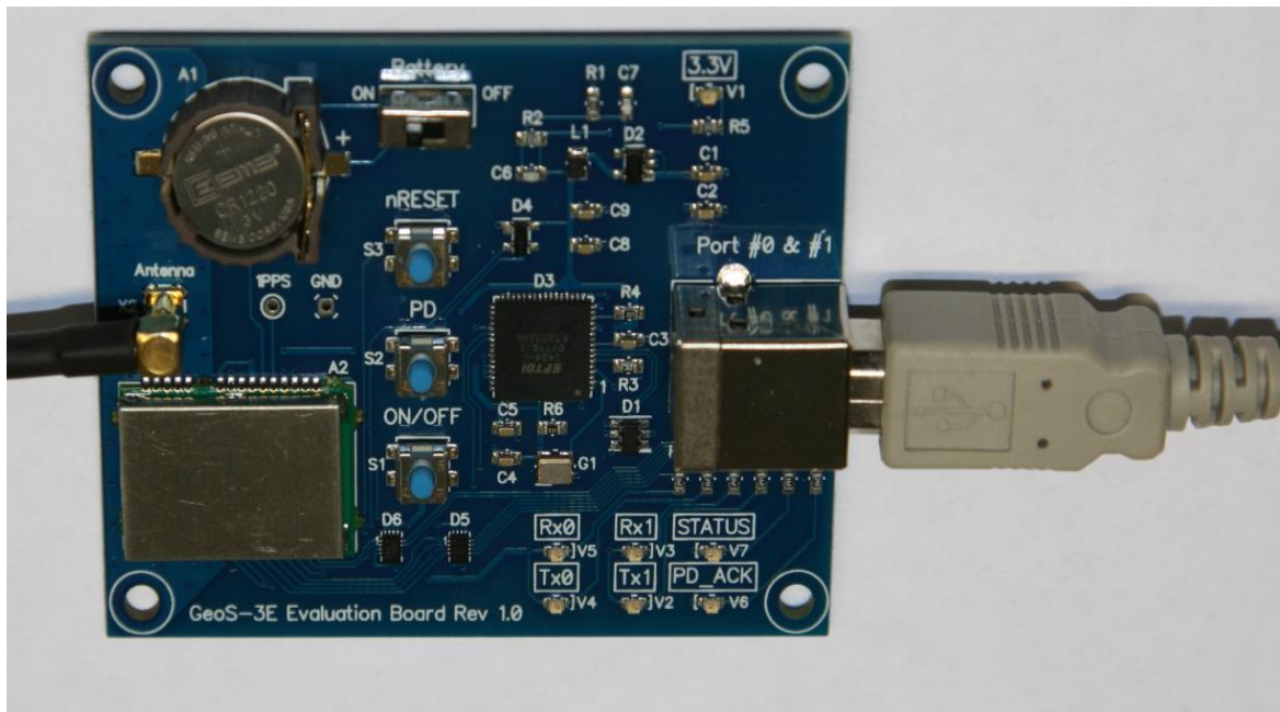
Рис. 4. Подключение антенны и USB порта
