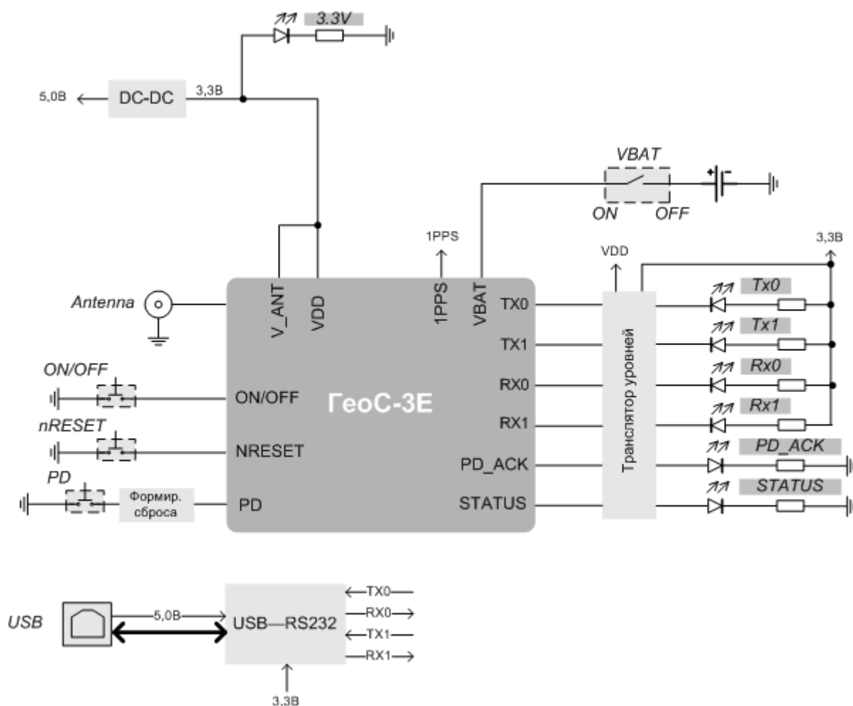
Рис. 2. Структурная схема платы
