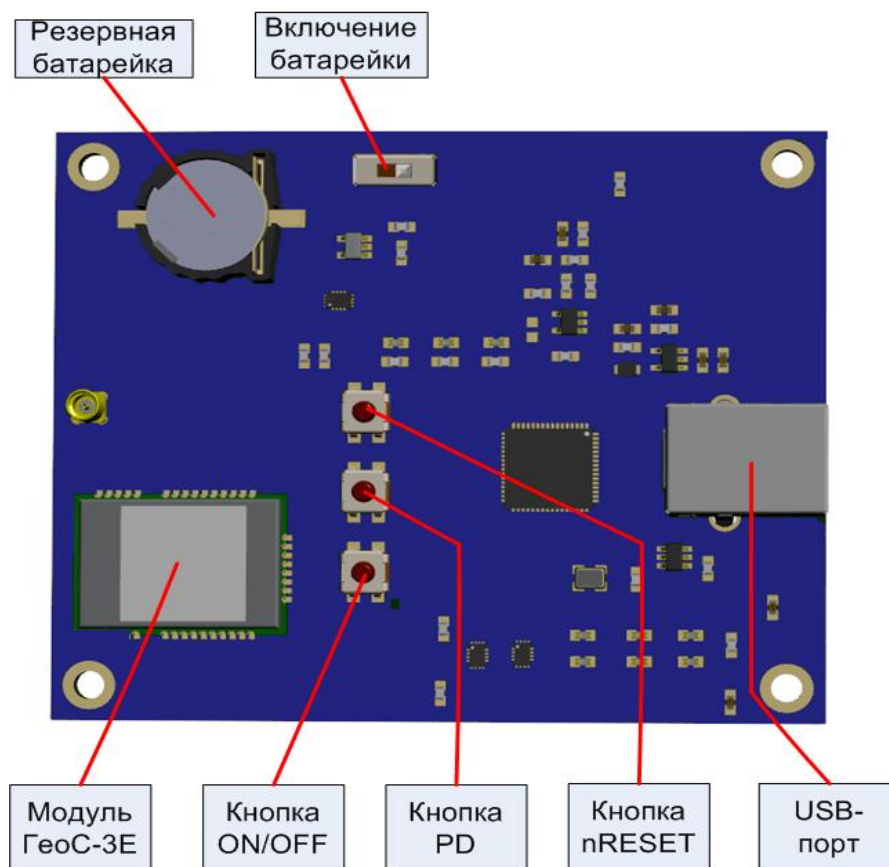
Рис. 1. Общий вид платы
