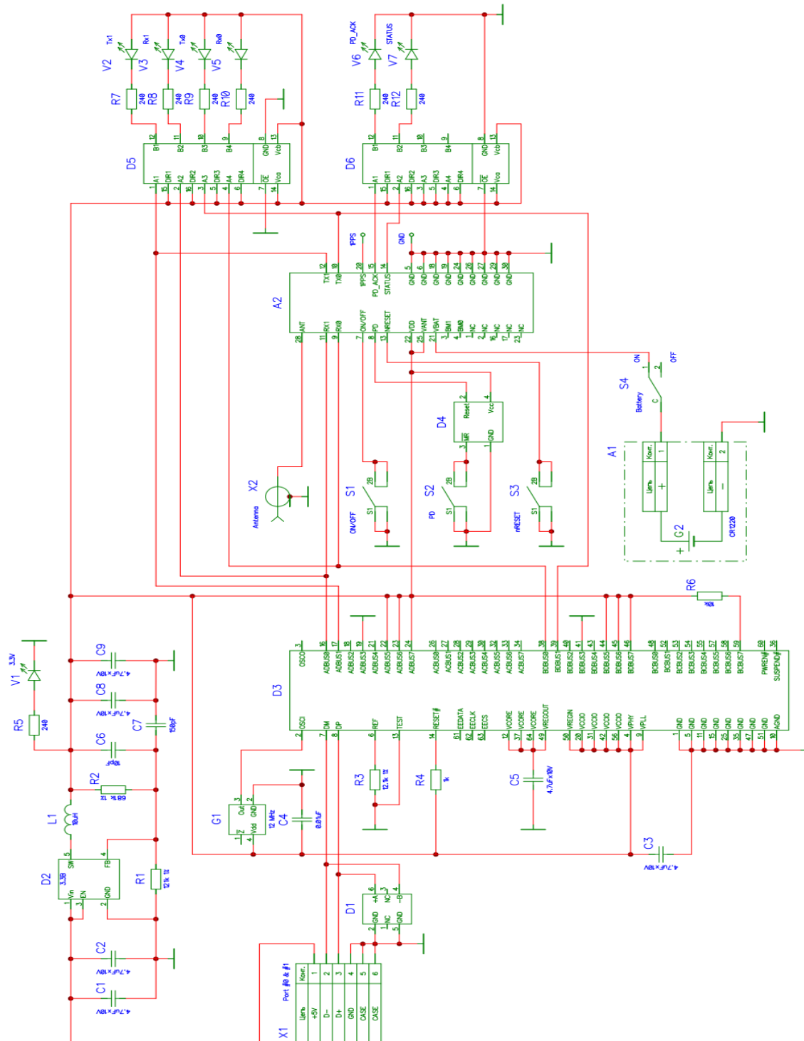
Рис. 5. Схема электрическая принципиальная
