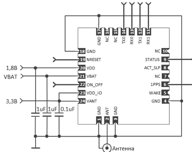
Рис. 9. Типовая схема включения модуля
