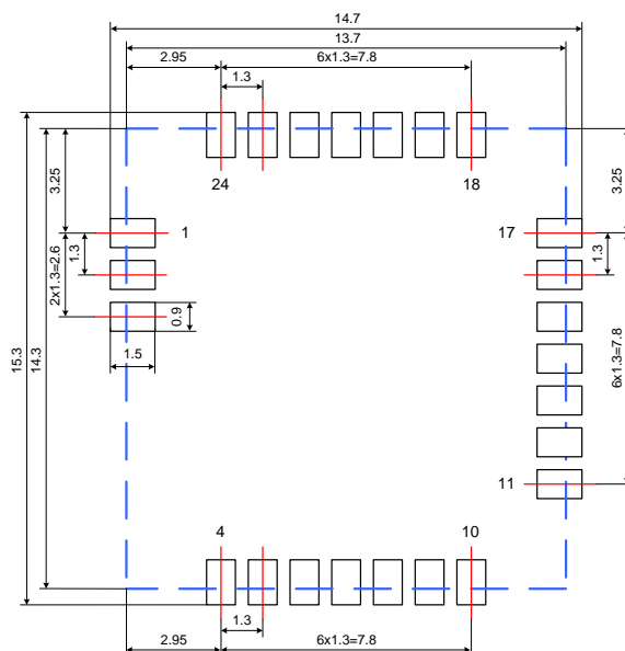
Рис. 6. Рекомендуемое посадочное место
