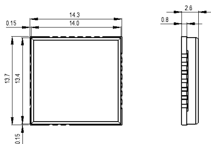
Рис. 4. Габаритный чертеж
