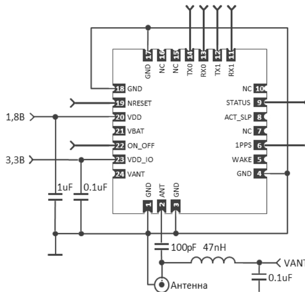
Рис. 10. Упрощенная схема включения модуля
