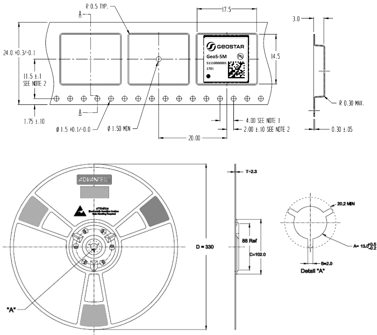
Рис. 8. Упаковка: в катушке – 1000 модулей
