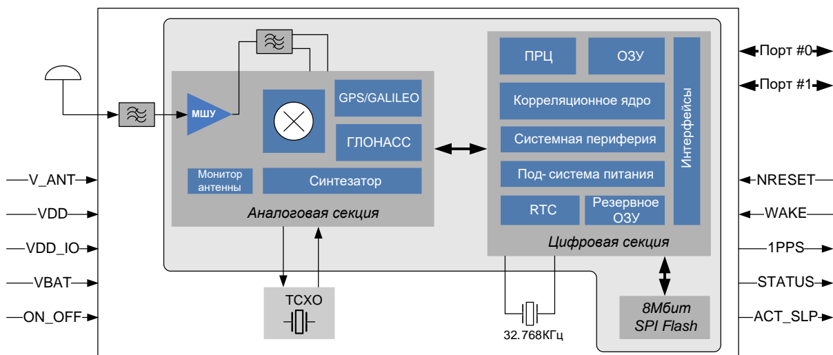
Рис. 1. Структурная схема
