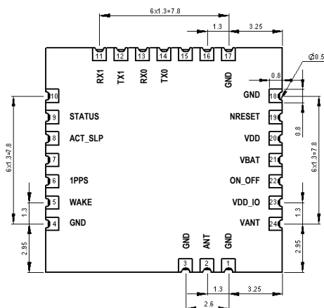
Рис. 5. Чертеж контактных площадок
