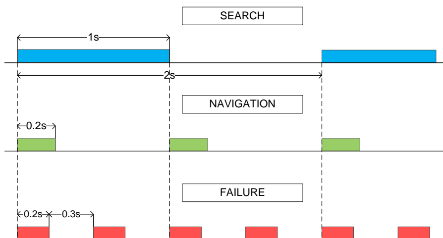
Рис. 2. Временные диаграммы на выводе STATUS
